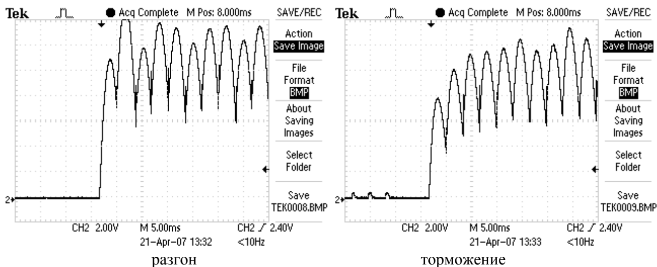
Рисунок 9-6 Кривые тока якоря с перерегулированием
