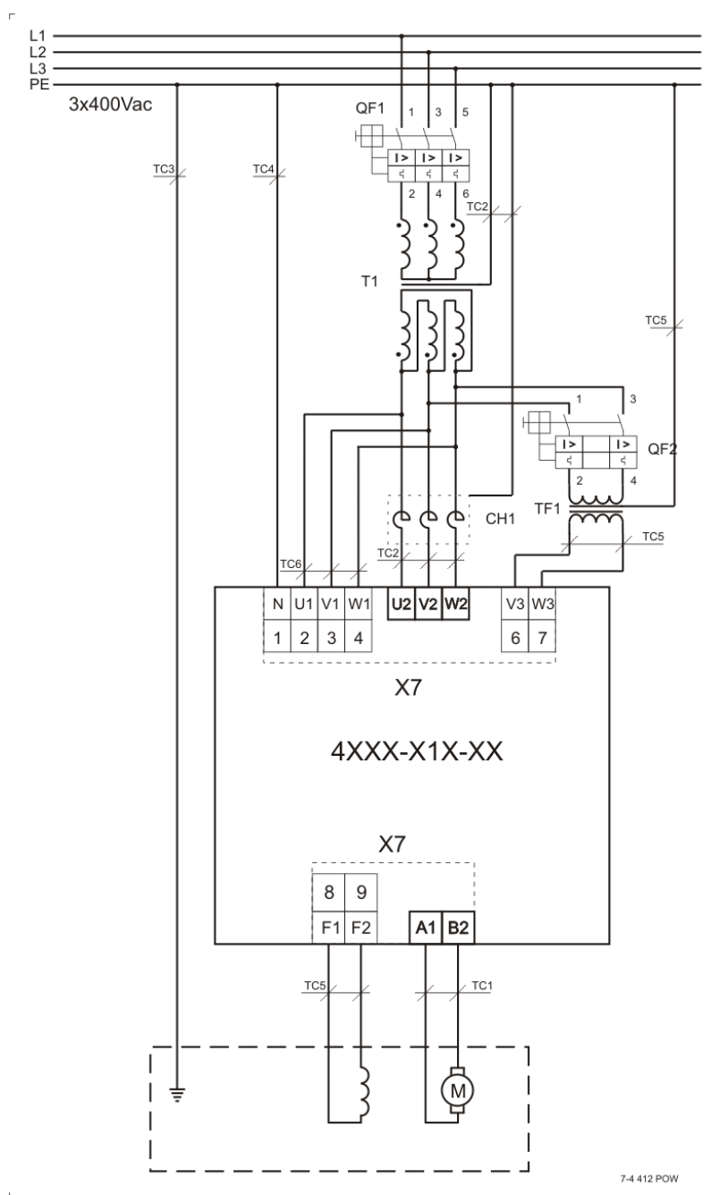
Рисунок 7-4 Схема подключения преобразователя с понижающим трансформатором
