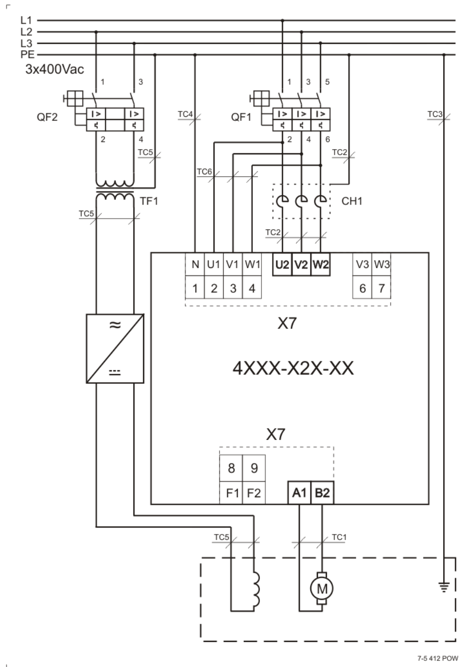
Рисунок 7-5 Схема подключения преобразователя с внешним возбуждением
