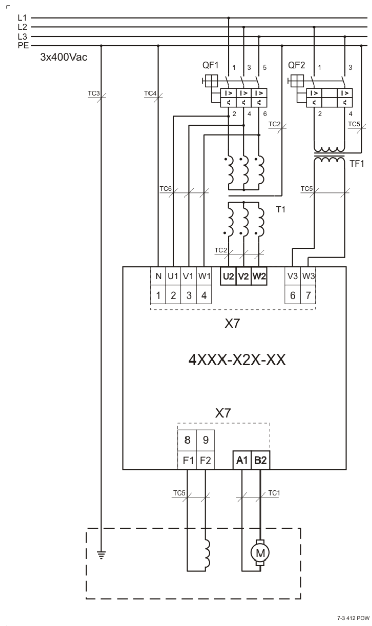
Рисунок 7-3 Схема подключения преобразователя с понижающим трансформатором
