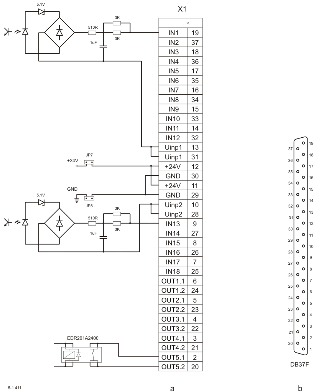
Рисунок 5-1 Соответствие между сигналами и выводами разъема параллельного интерфейса X1 и принципиальные схемы цифровых входов и выходов
